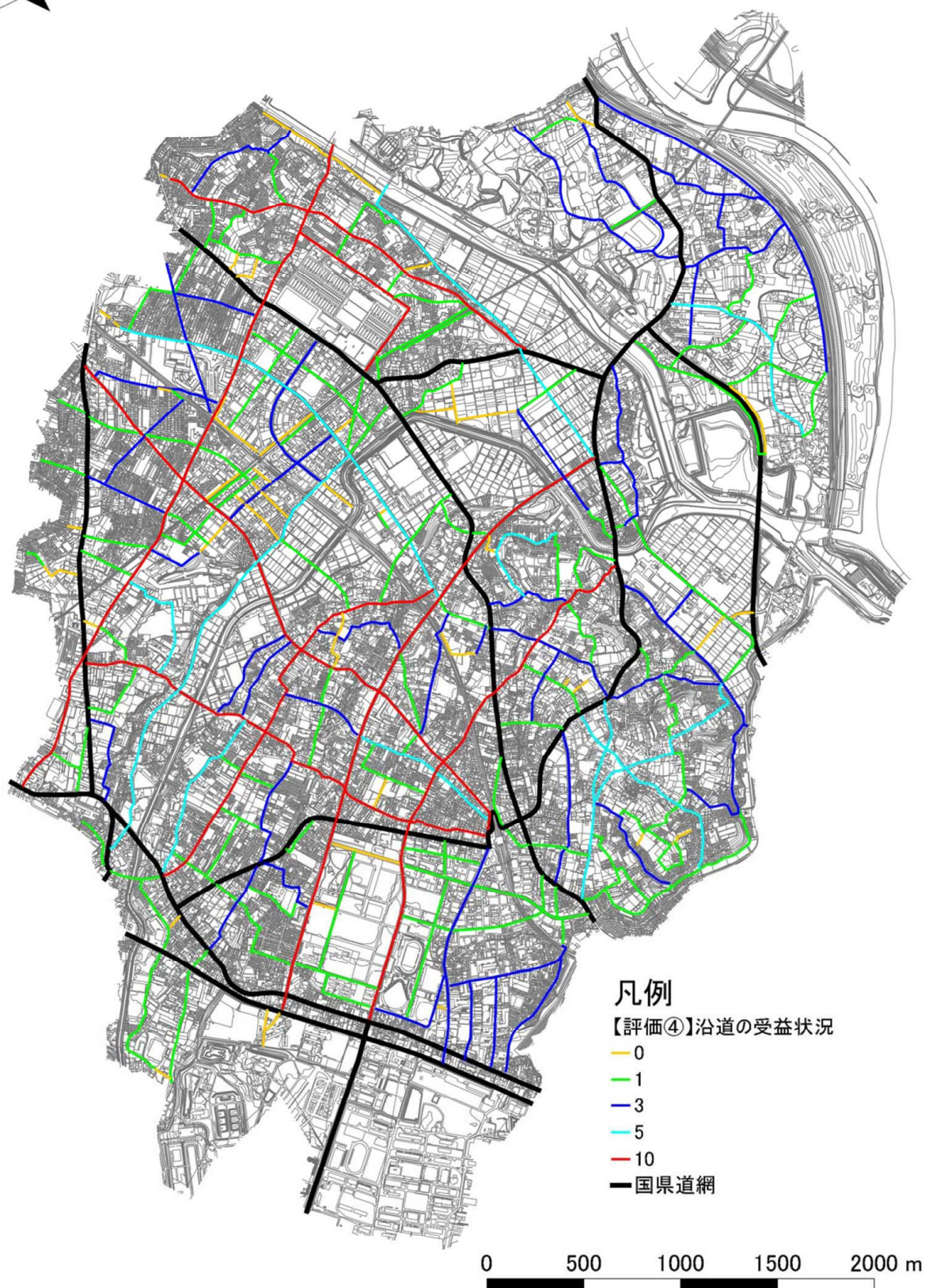
図6-4 道路網図【評価④】
