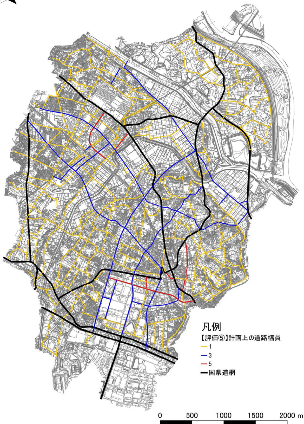
図6－5 道路網図【評価⑤】
