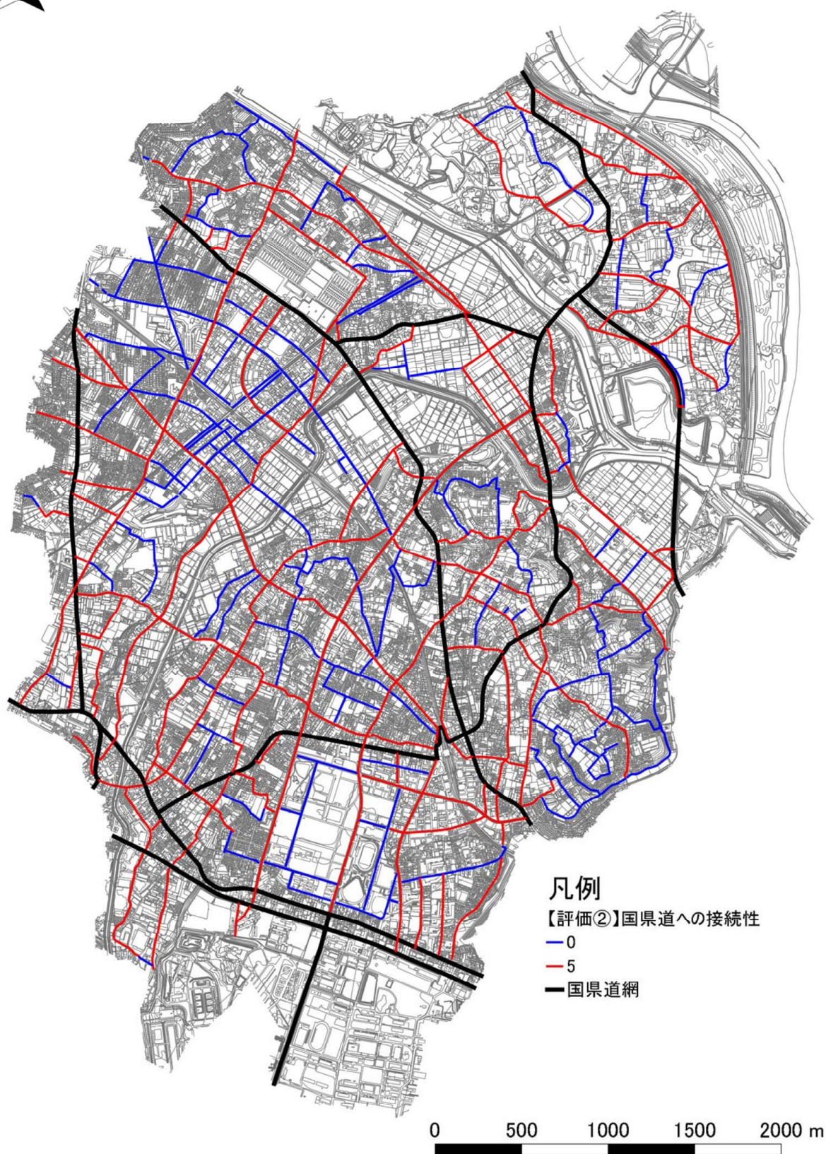
図6-2 道路網図【評価②】
