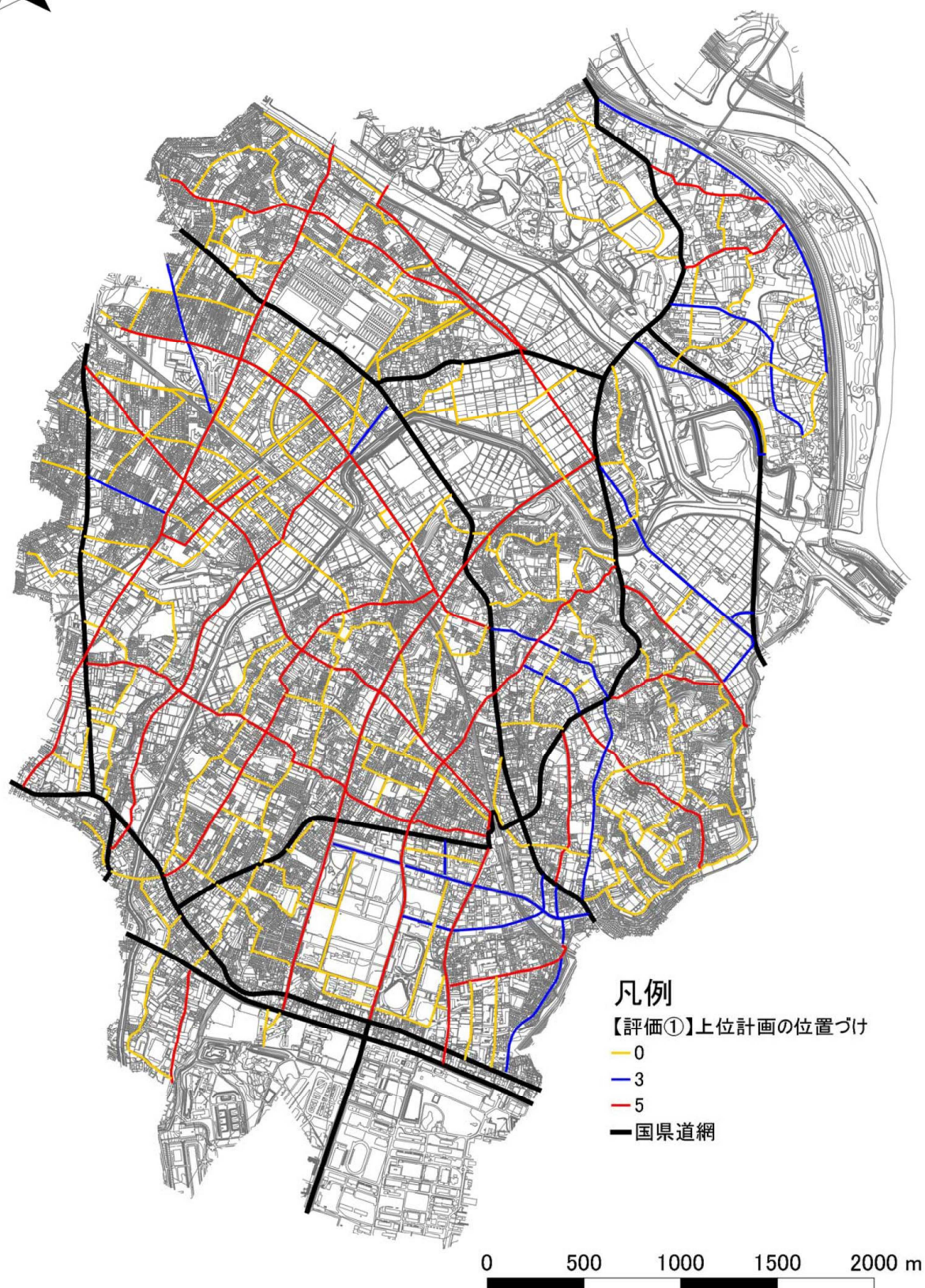
図6-1 道路網図【評価①】
