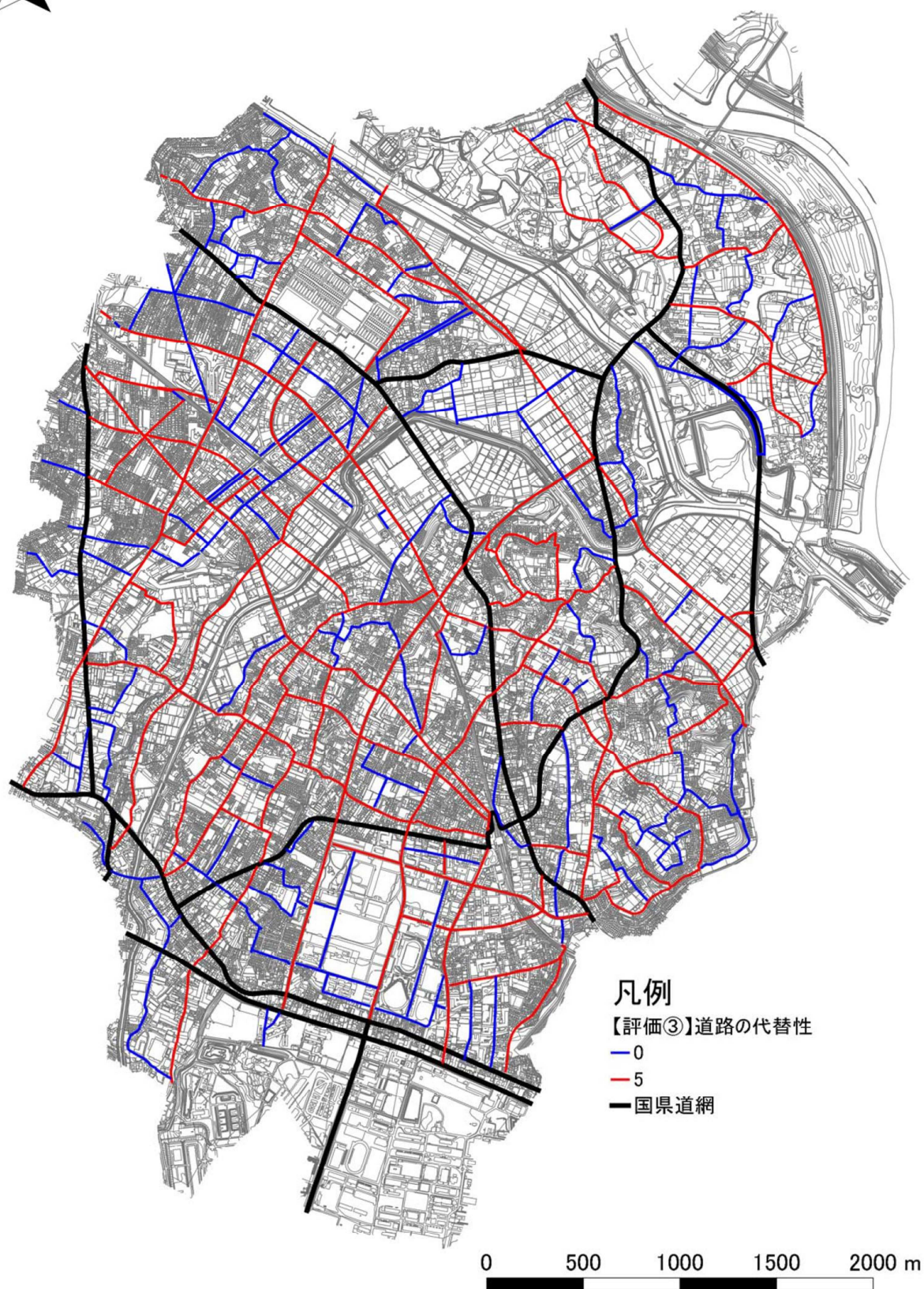
図6-3 道路網図【評価③】
