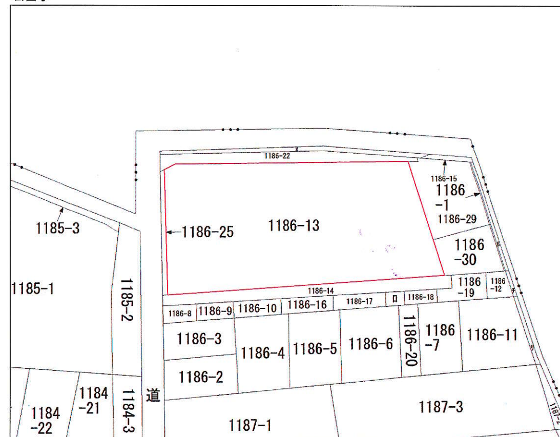
公図写
