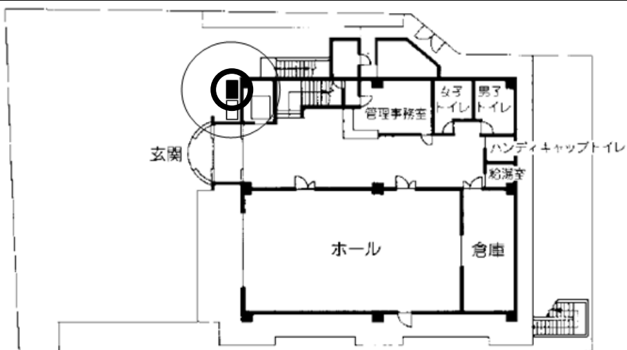
平面図
