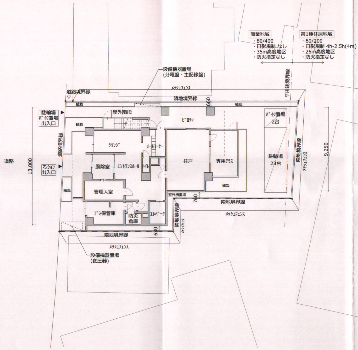
1階平面図 兼 土地利用計画図
