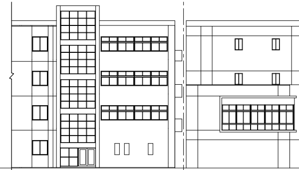
西立面图 S=1:400
