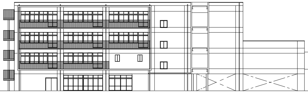
北立面图 S=1:400
