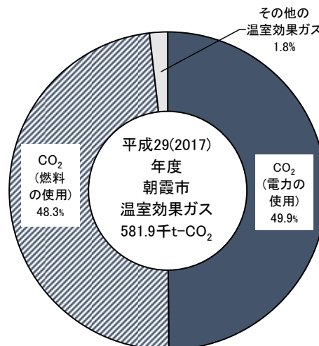
■温室効果ガス排出量の内訳
