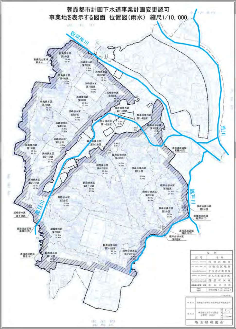
出典：荒川右岸流域関連朝霞公共下水道 事業計画変更協議申出書 平成30年度 図 2-1 下水道計画一般図（雨水）
