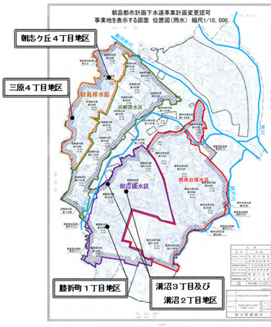
出典：荒川右岸流域関連朝霞公共下水道 事業計画変更協議申出書 平成30年度 図 4-2 排水区別位置図
