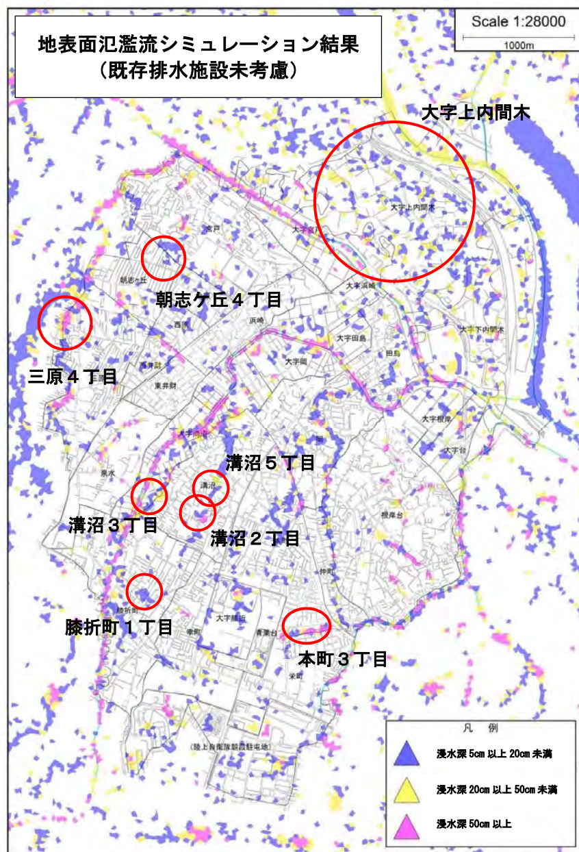
図 3-9 地表面氾濫流シミュレーション結果（既存排水施設未考慮）
