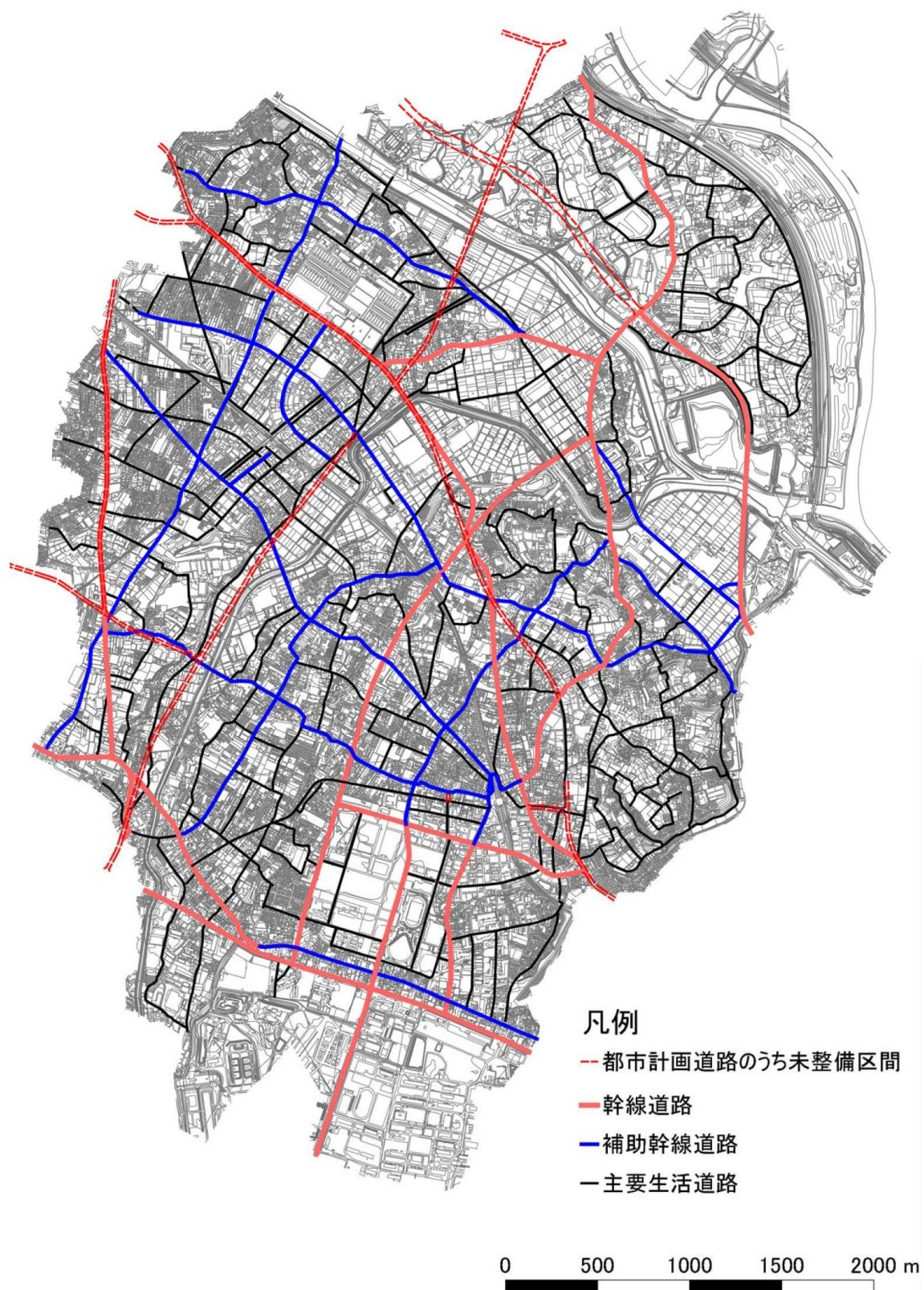
図5-1 目指すべき道路網図
