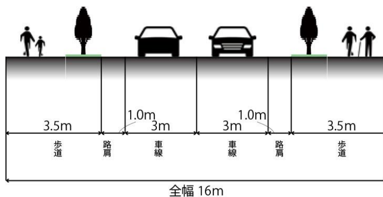
図4-2 標準断面モデル【幹線道路】
