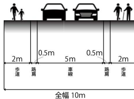
図4-3 標準断面モデル【補助幹線道路】
