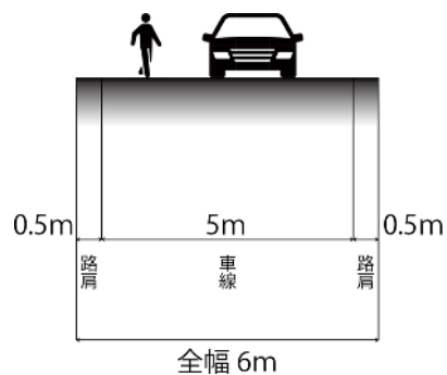
⑧【道路幅員 6mの場合】
