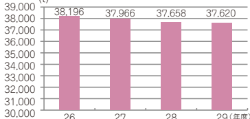
朝霞市のごみ総排出量推移
