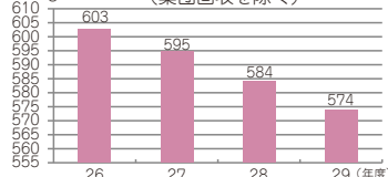
朝霞市の家庭ごみ1人1日排出量推移（集団回収を除く）
