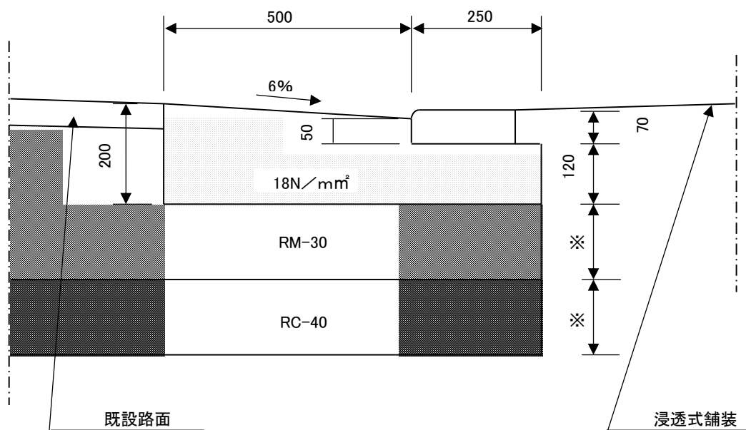
H-H'断面図
