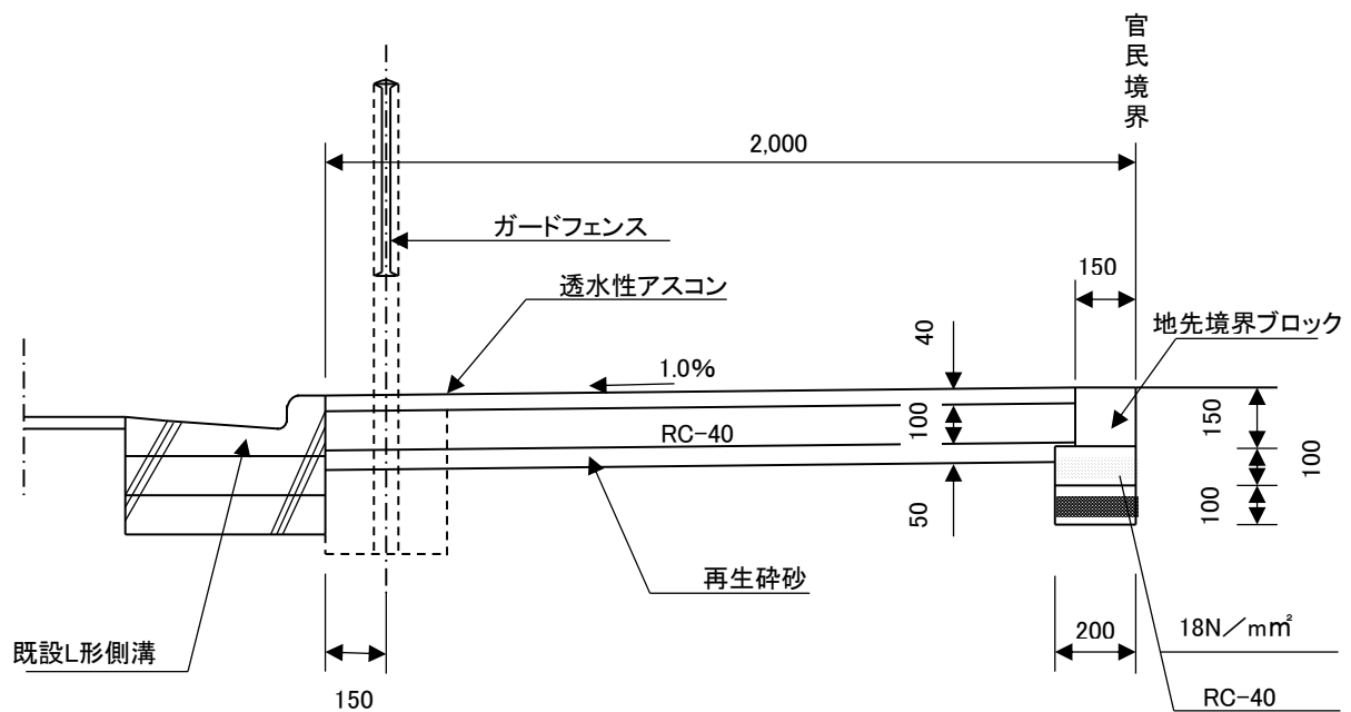
A-A'断面図
