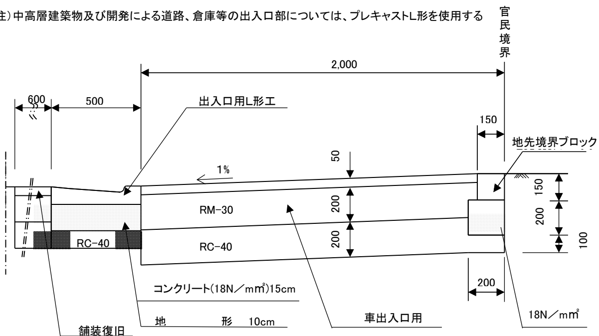
B-B'断 面 図
