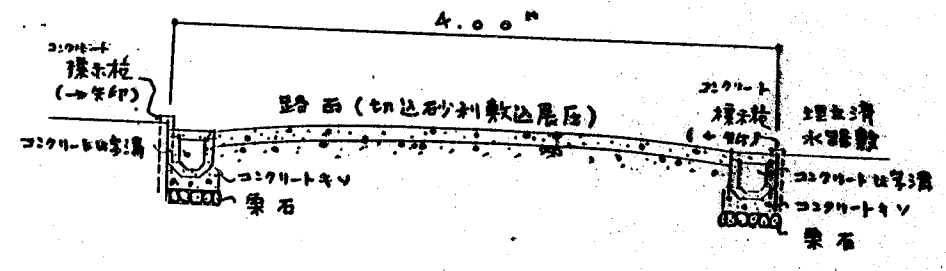
構造断面図 S=1:50
