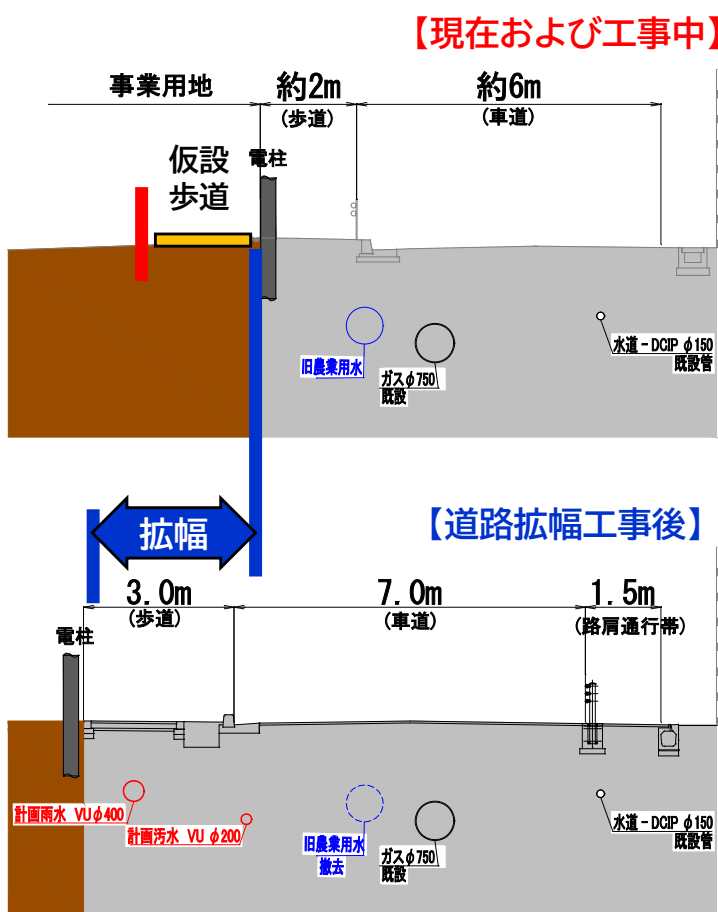
図2 市道6号線横断図 (上図:現在および工事中、下図:道路拡幅工事後)
