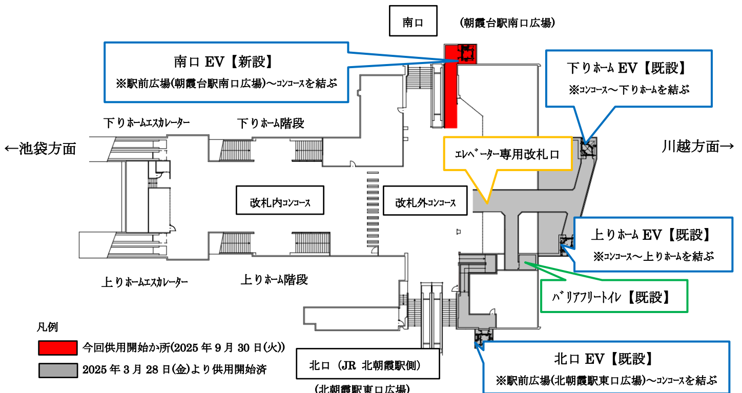
△朝霞台駅 改札階平面図（配置計画）
