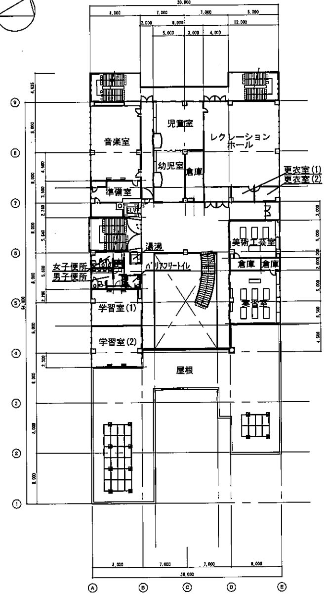
2階平面図 S=1/200
