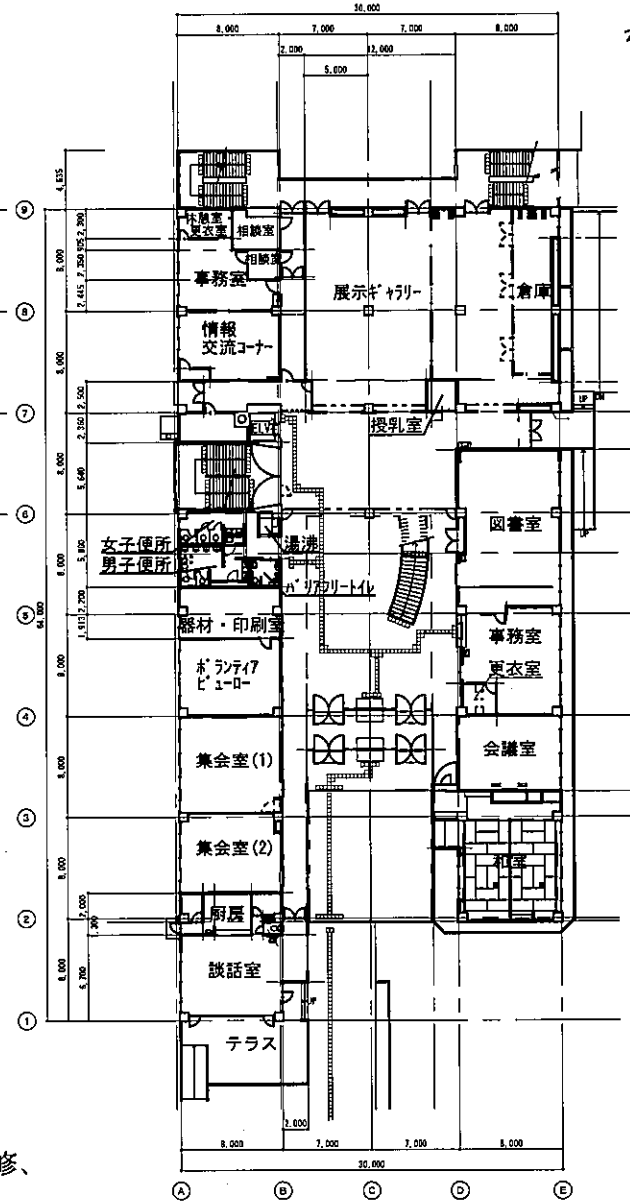
1階平面図 S=1/200
