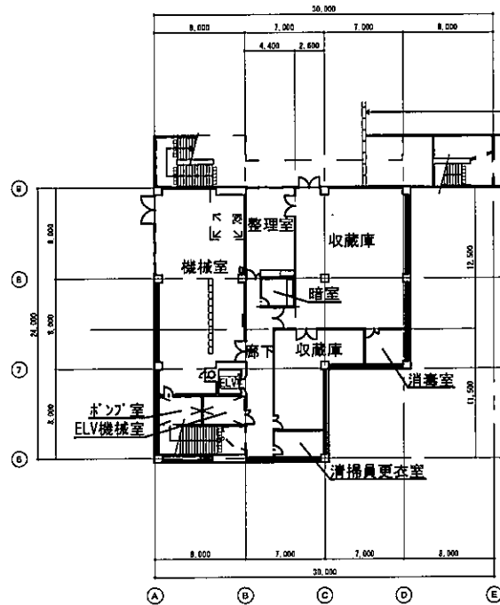
地階平面図 S=1/200
