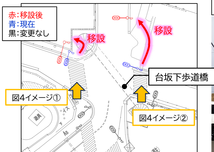
図3 信号機の移設箇所(2基)
