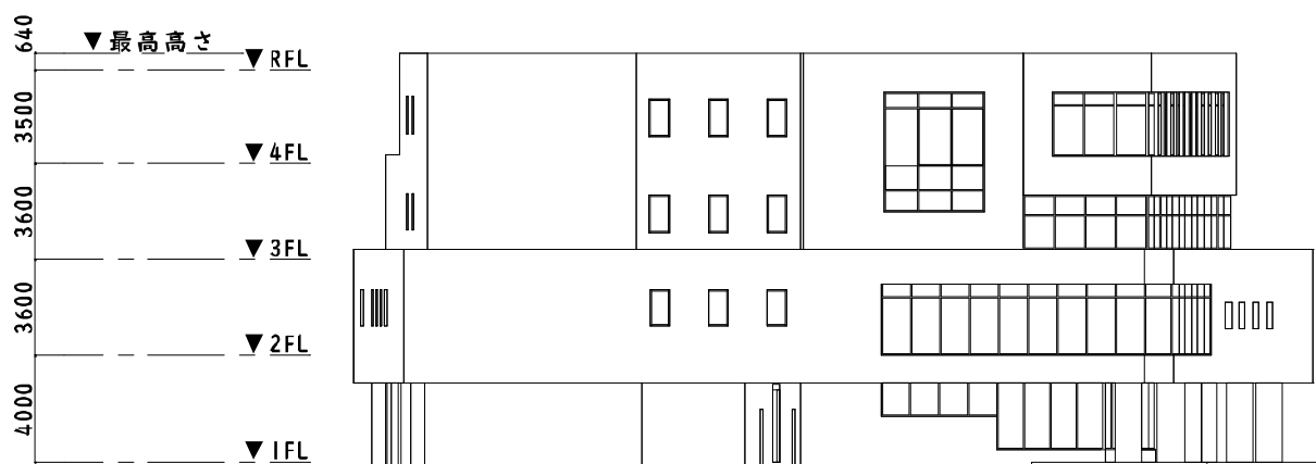
南西立面图
